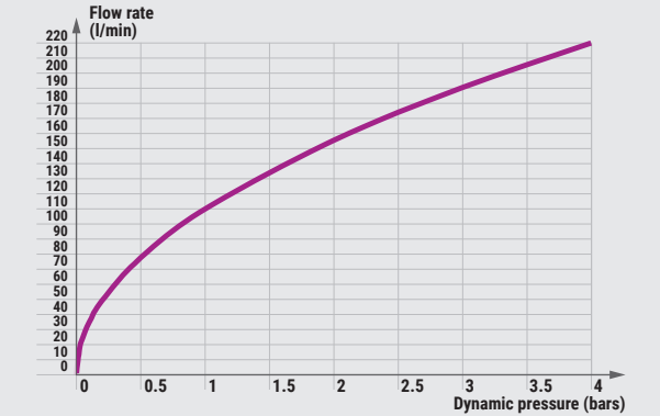
PRESTO 84009
