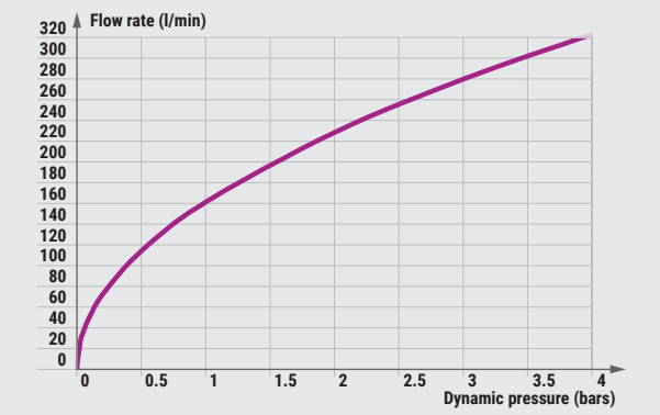
PRESTO 84020
