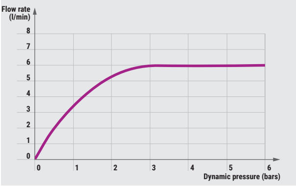
SENSAO® 5100 – 5200 – 5300
