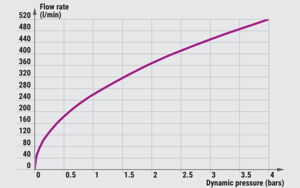
PRESTO 84021
