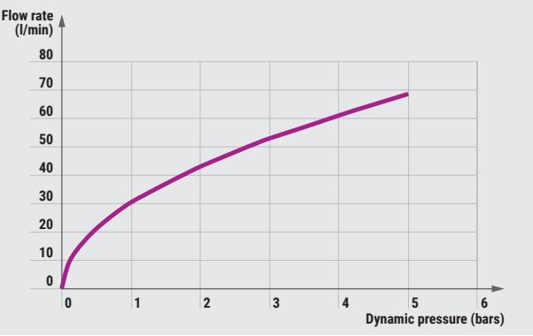
PRESTO 60 / 60 B
