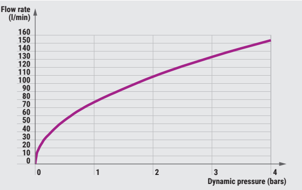
PRESTO 84008
