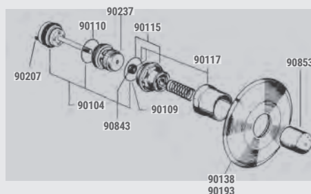
PRESTO 50 / 50 B
